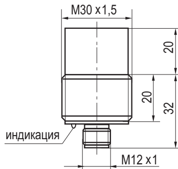
Габаритный чертеж
